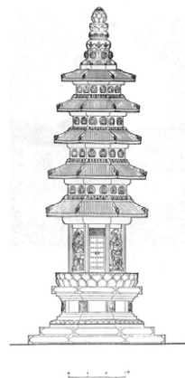
圖 10 棲霞寺舍利塔立面圖（圖片來源：劉敦楨《中國古代建築史》）
