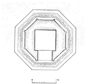
圖 9 棲霞寺舍利塔平面圖（圖片來源：劉敦楨《中國古代建築史》）
